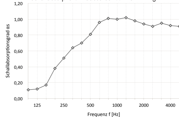
Schallabsorption: Bildabsorber WILDSPITZE light
